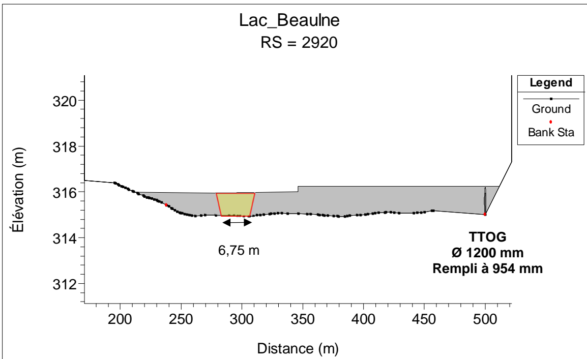
Barrage du lac intermédiaire et sa brèche avec le débit de récurrence 1000 ans modélisé dans HEC-RAS
