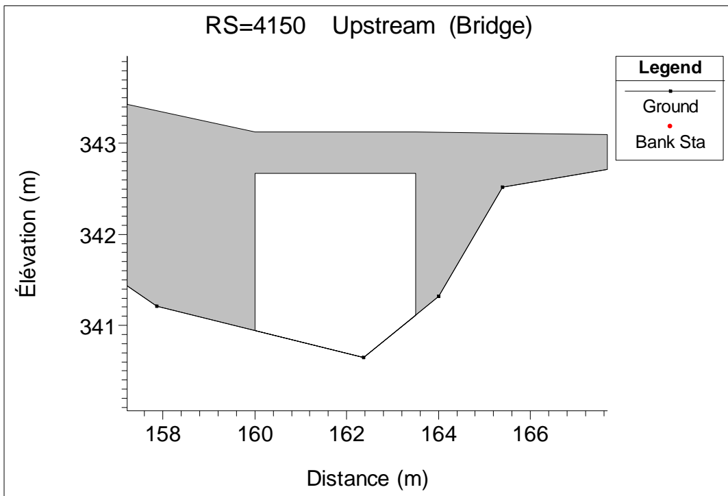
Pont de la section 4150 modélisé dans HEC-RAS
