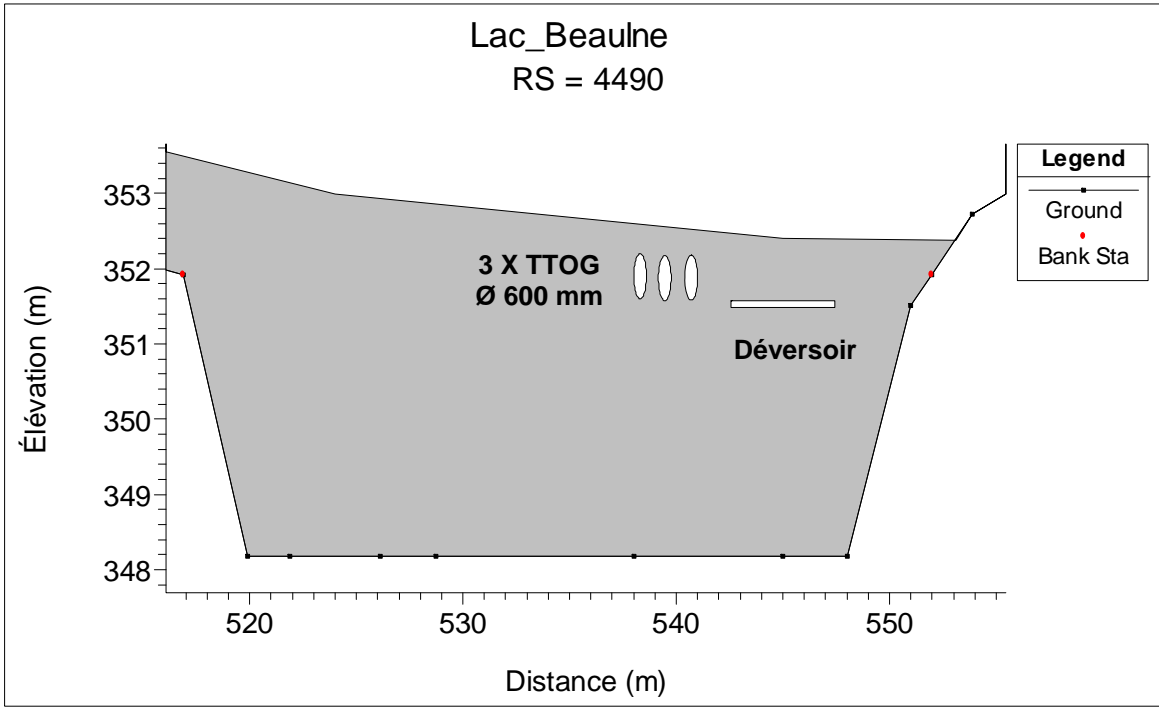
Barrage du lac Beaulne modélisé dans HEC-RAS
