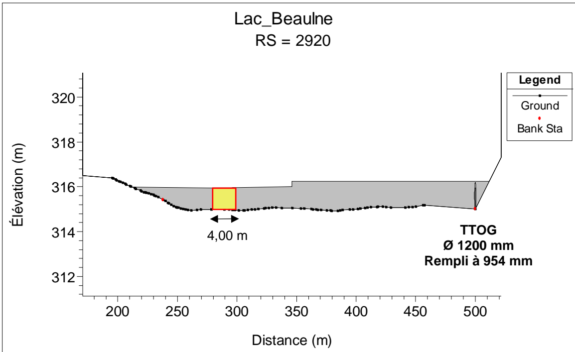
Barrage du lac intermédiaire et sa brèche avec le débit module modélisé dans HEC-RAS
