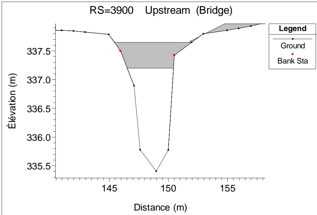
Pont de la section 3900 modélisé dans HEC-RAS
