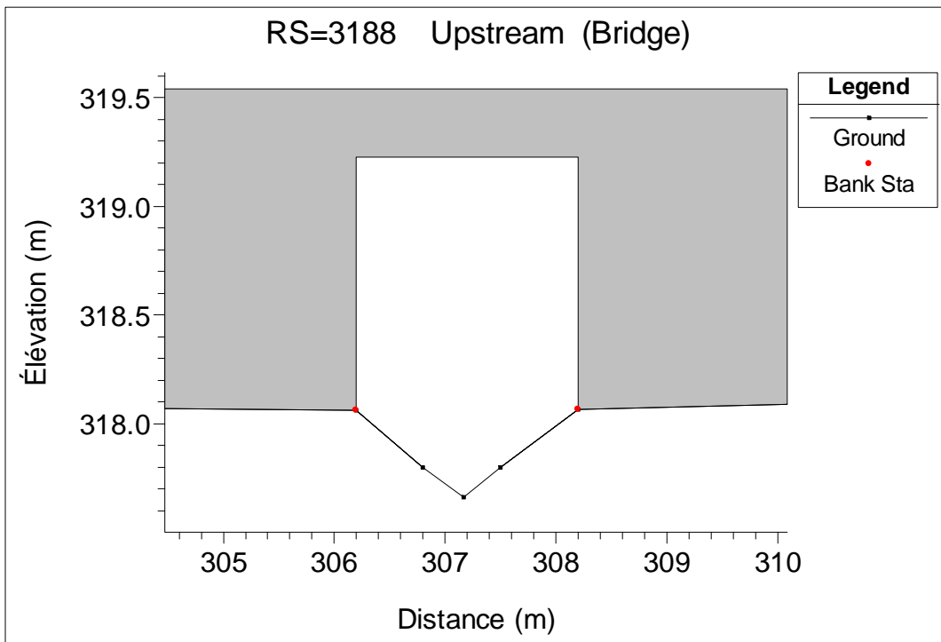
Pont de la section 3188 modélisé dans HEC-RAS
