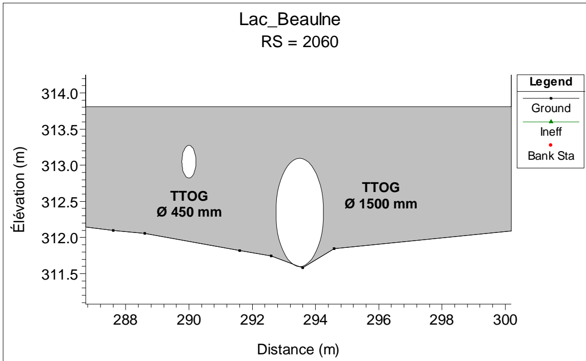
Ponceau du chemin Cordon de Chertsey modélisé dans Hec-Ras
