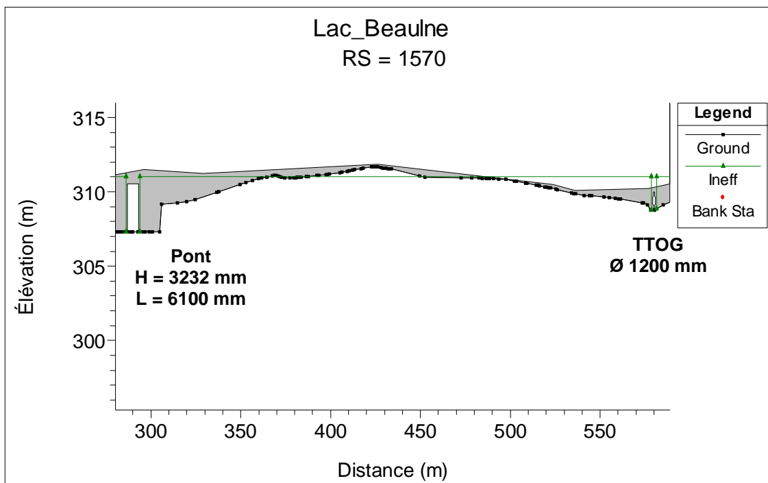
Pont et ponceau de l'île du lac Duffy modélisés dans Hec-Ras
